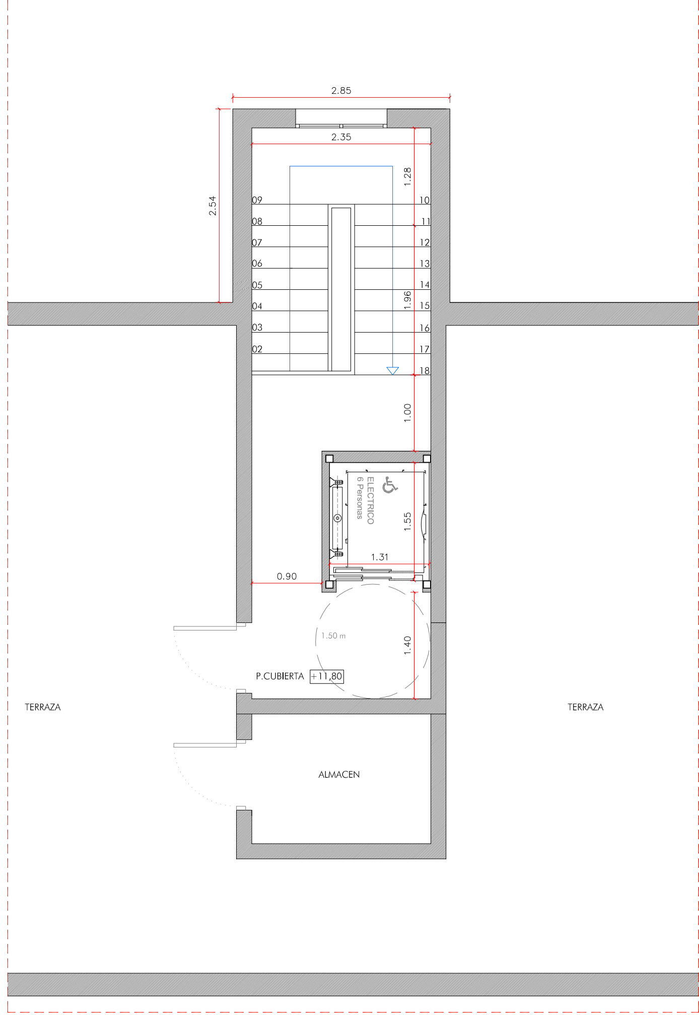
Planta Cubierta E 1:50
