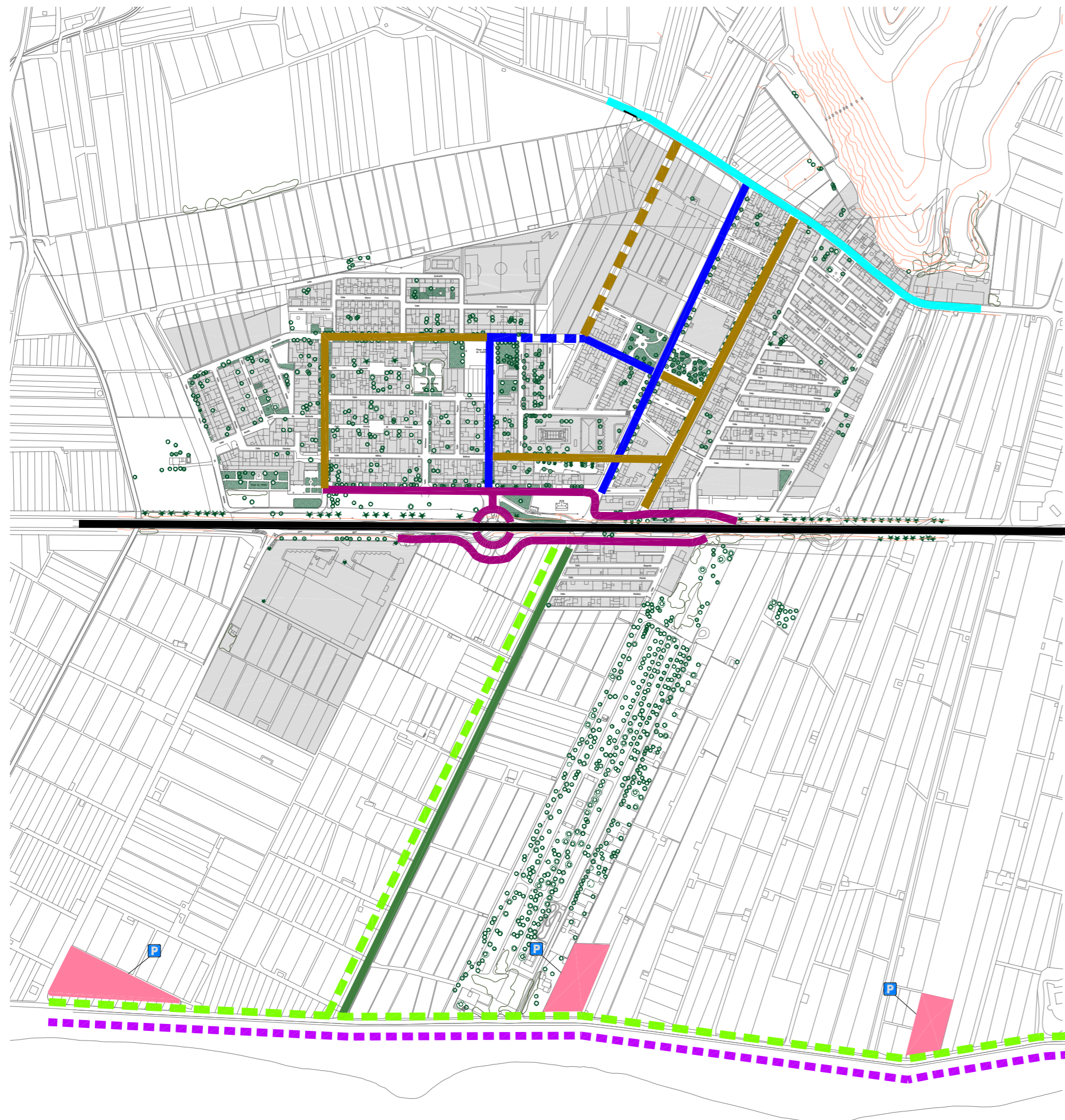
Estructura viaria
